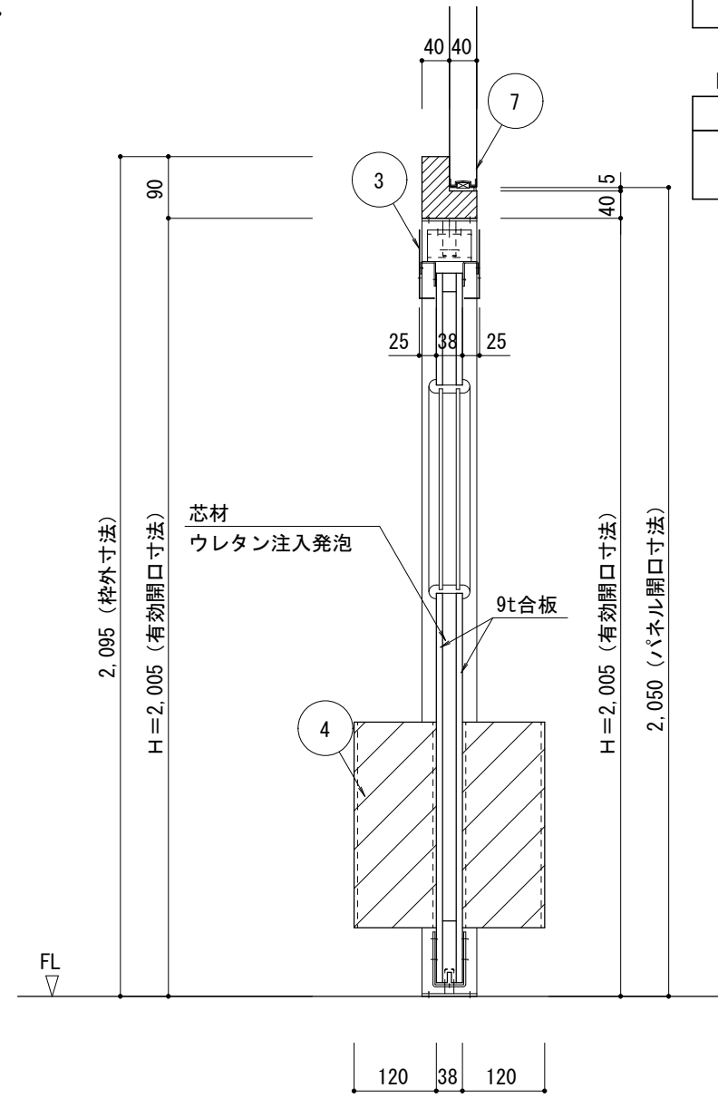
断面図 S=1/10
