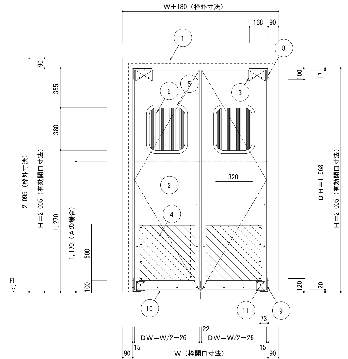
立面図 S=1/20
