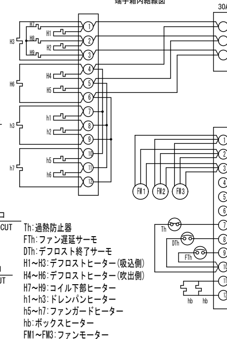
端子箱内結線図
