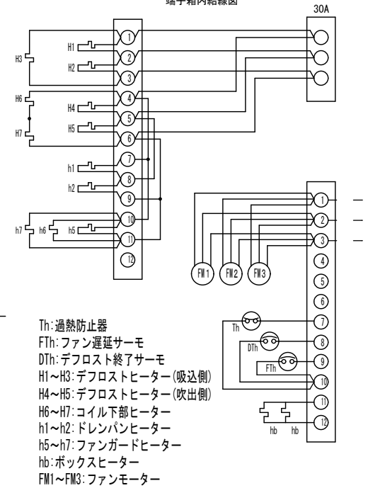
端子箱内結線図
