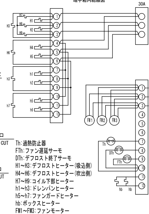
端子箱内結線図
